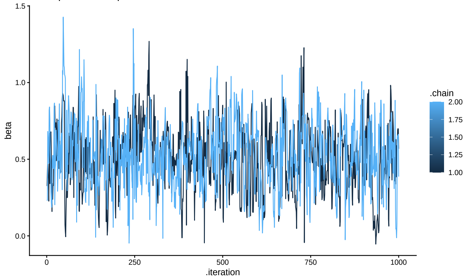
Trace plot for beta parameter
